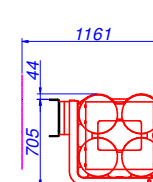
Sezione A-A
