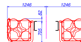
Sezione A-A
