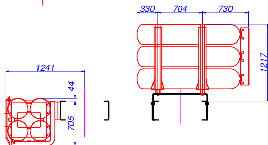
Sezione A-A
