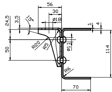
Section A-A(B-7) Scale: 1:2
