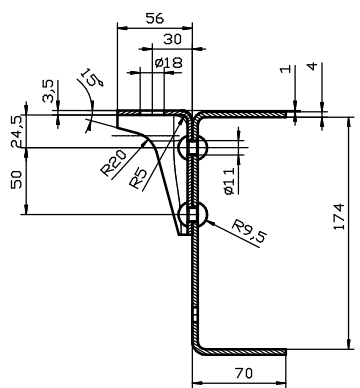
Section A-A(B-7) Scale: 1:2
