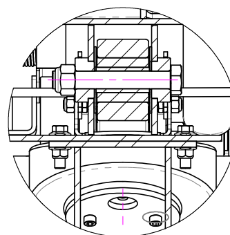
SEZIONE A-A SCALA 1 : 5
