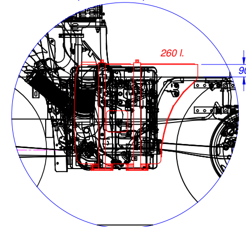
Serbatoio da 260 litri (cod. 05019074) (in alternativa)
